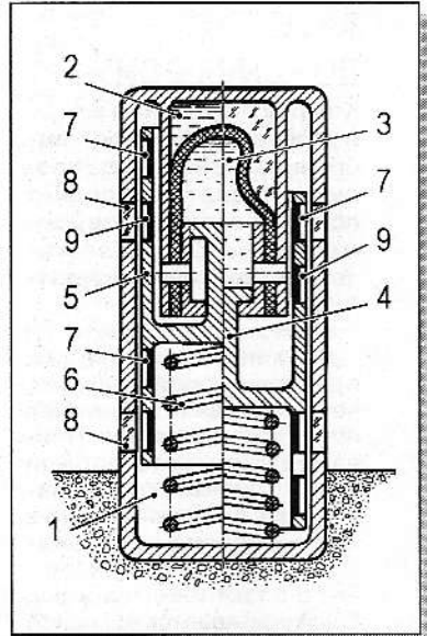
Сигнализатор гололеда. Разрез.
